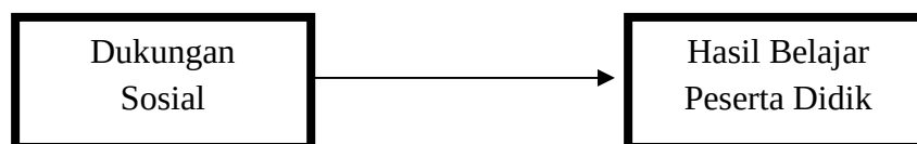
Gambar 2.2 Kerangka Teoritik
